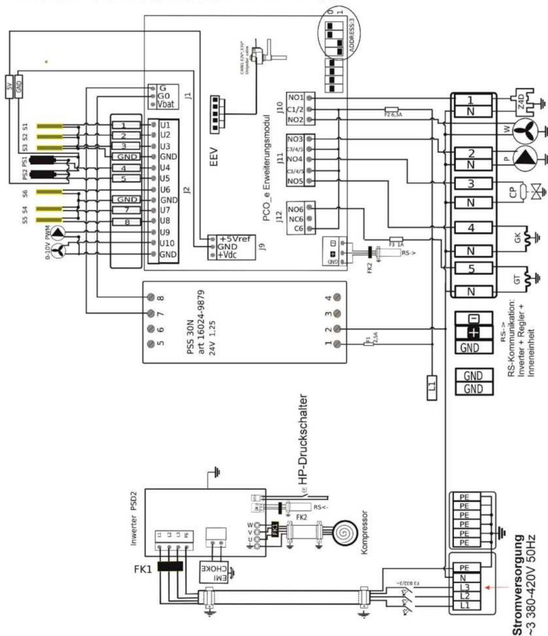
Abbildung 13: Elektrischer Schaltplan der Steuerung
