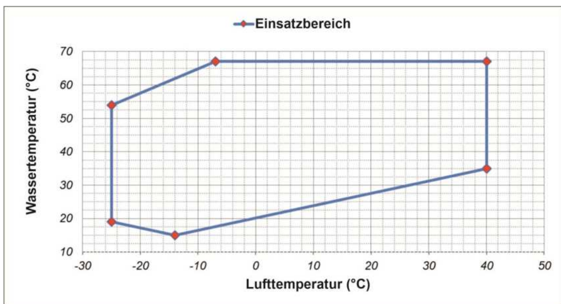
Abbildung 15: Einsatzbereich Schema
