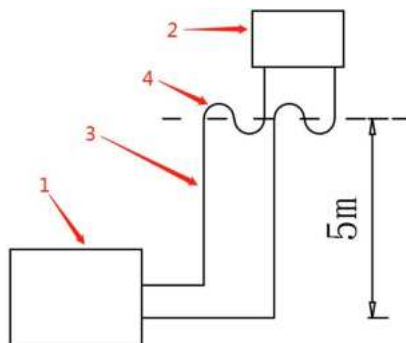
Anschlusschema, wenn das Innengerät oben steht
