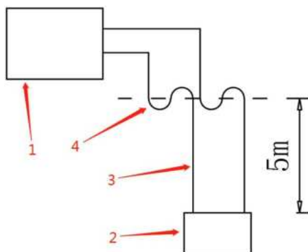
Anschlusschema, wenn das Innengerät oben steht
